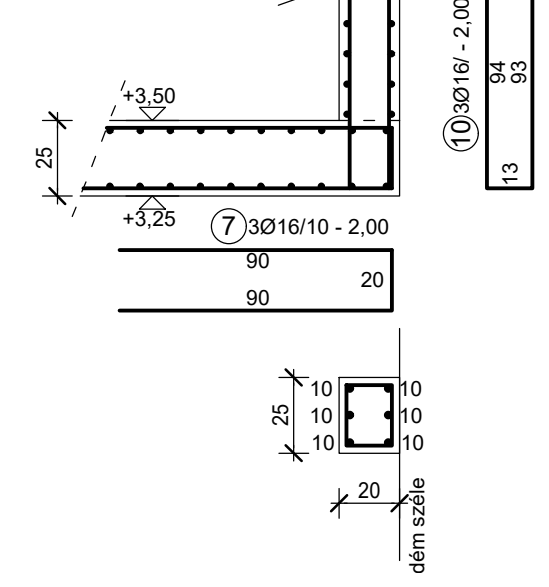
Monolit pillér [MP1;MP2] tűskézése M=1:25
