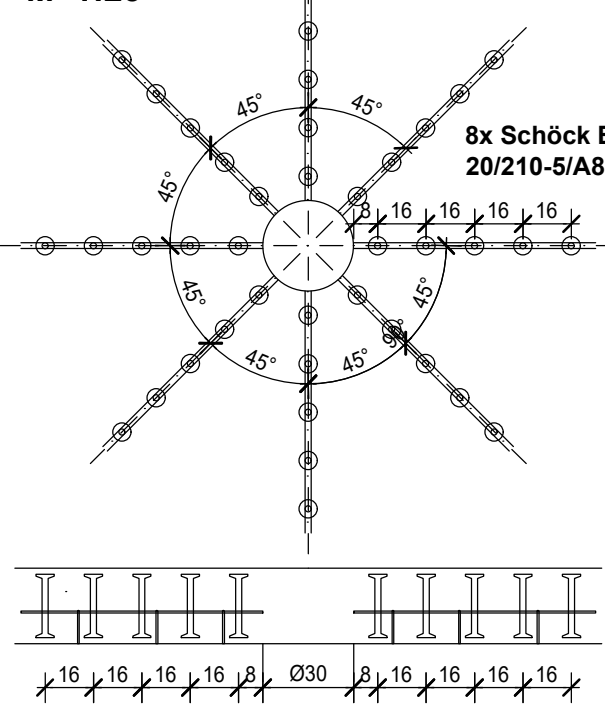
Átszuródási vasalás elhelyezése általános helyen M=1:25
