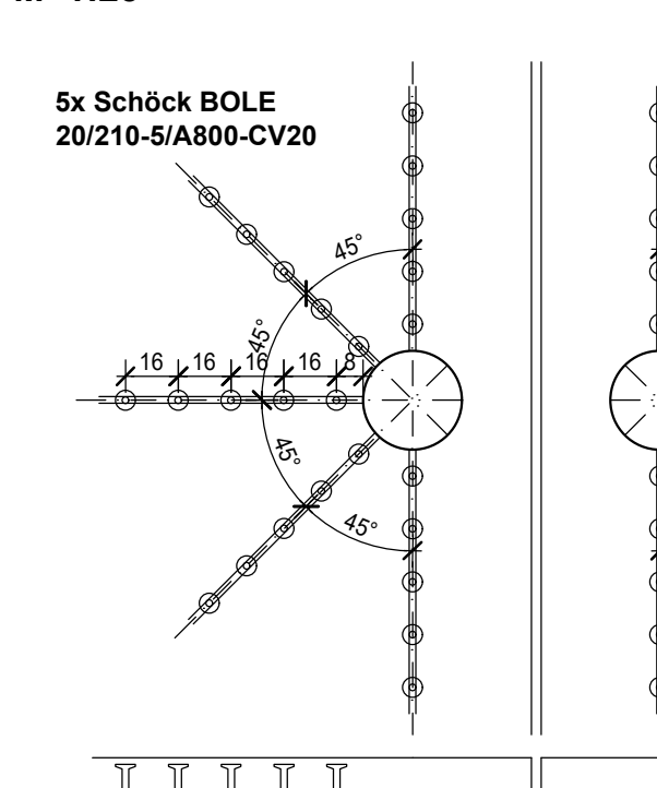
Átszuródási vasalás elhelyezése a dilatációnál (11*;11* raszterek) M=1:25
