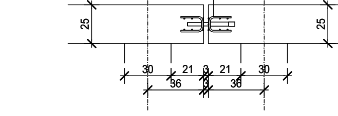
Dilatáció kialakítása M=1:25
